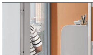
Zusätzliche Stahlbolzen zwischen Türblatt und Zarge gegen Aufhebeln!
